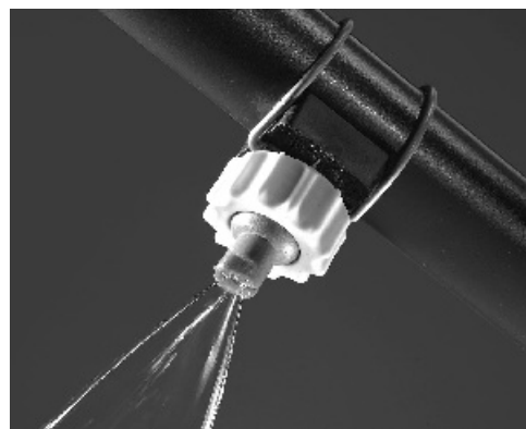
Boor een gat van 14,5 mm. in de leiding om de klembeugel te kunnen monteren.
